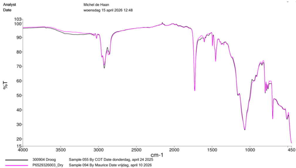
Spectra 1: Vergelijking droog C227303 F2600324
