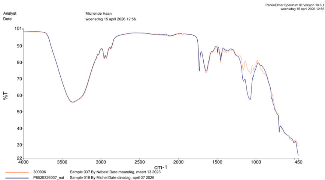
Spectra 2: Vergelijking nat C227304 F2600434
