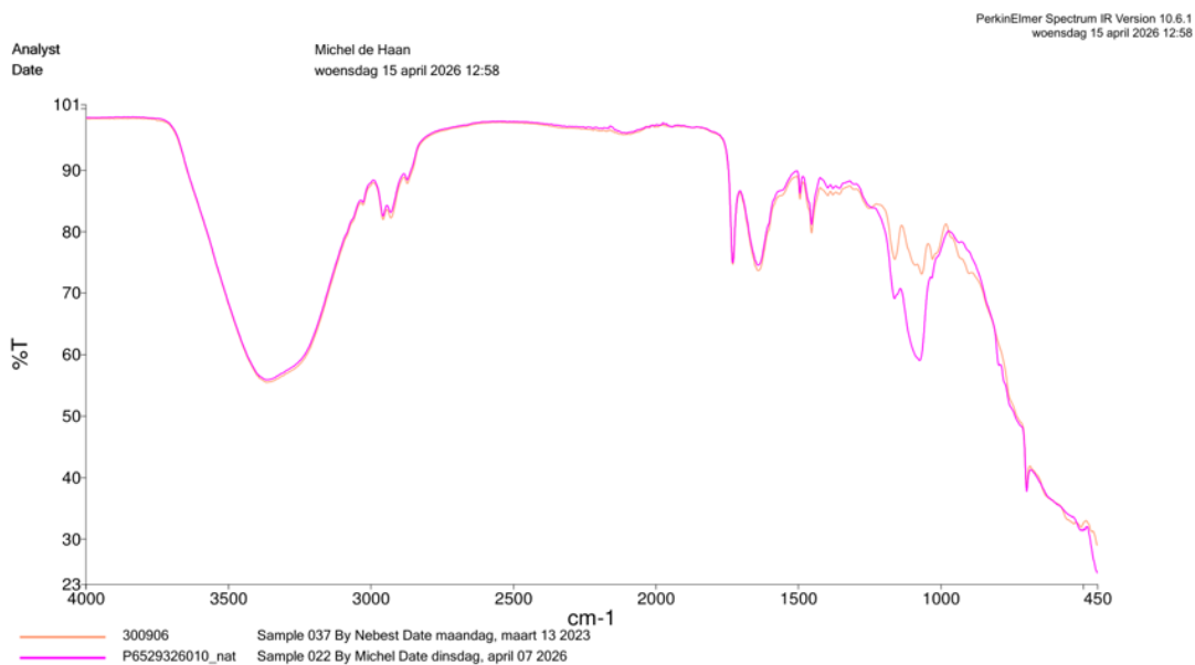
Spectra 2: Vergelijking nat C227304 F2600437
