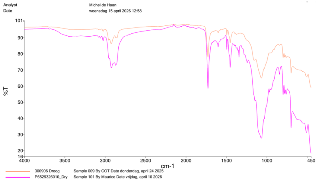
Spectra 1: Vergelijking droog C227304 F2600437
