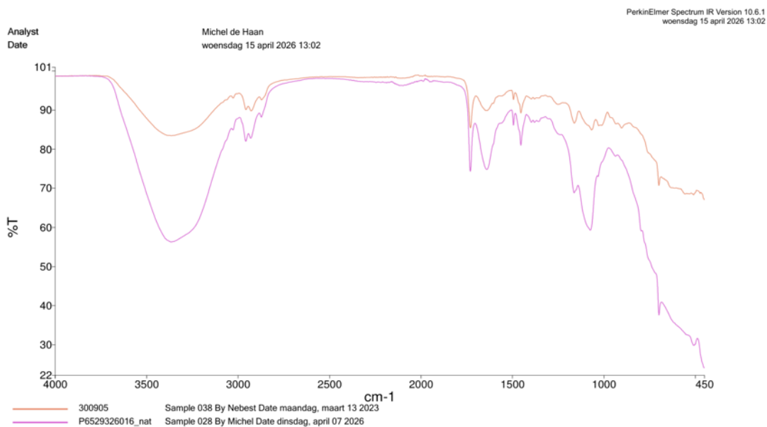
Spectra 2: Vergelijking nat C227307 F2600441
