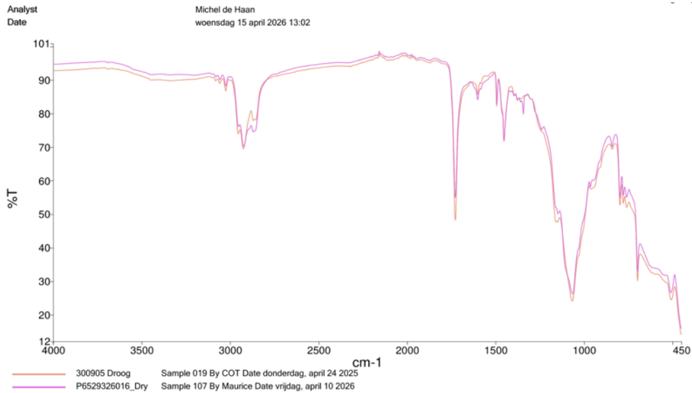
Spectra 1: Vergelijking droog C227307 F2600441
