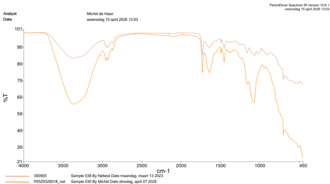
Spectra 2: Vergelijking nat C227307 F2600443
