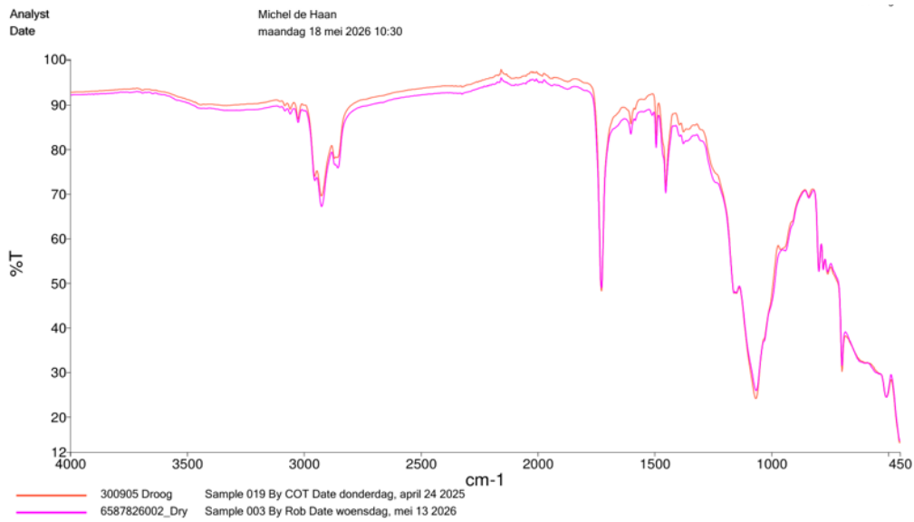
Spectra 1: Vergelijking droog C227306 F2600835
