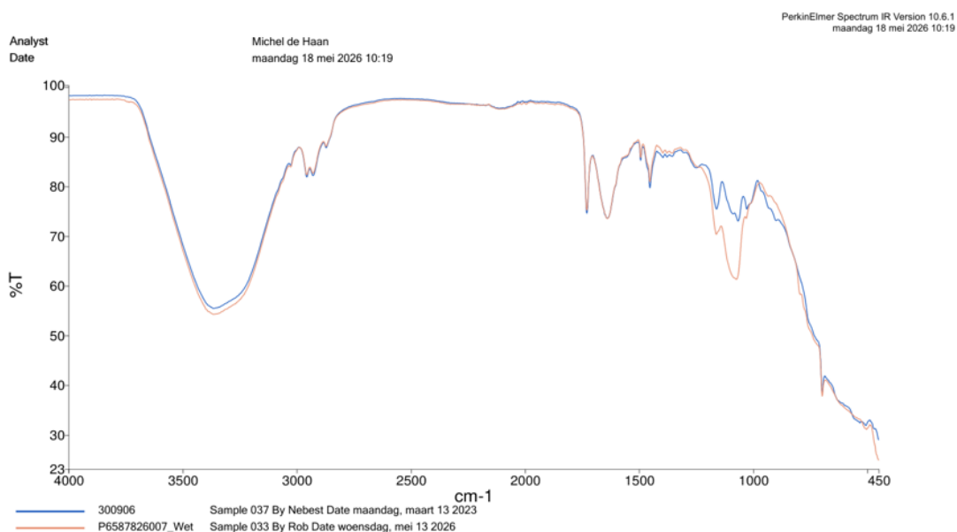
Spectra 2: Vergelijking nat C227304 F2600689
