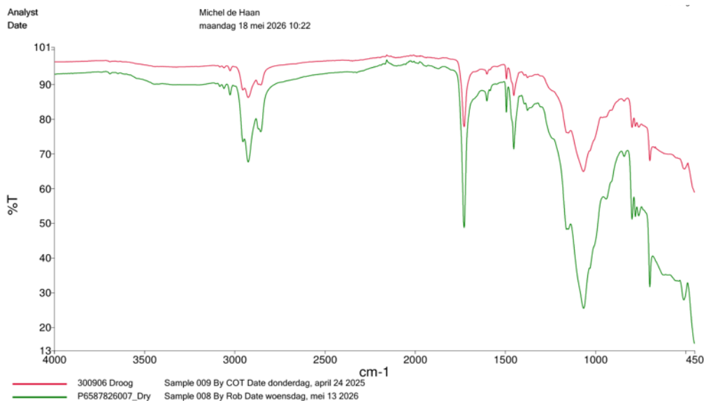
Spectra 1: Vergelijking droog C227304 F2600689
