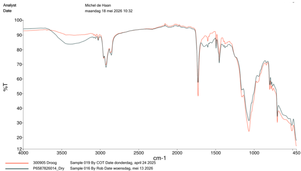
Spectra 1: Vergelijking droog C227307 F2601091
