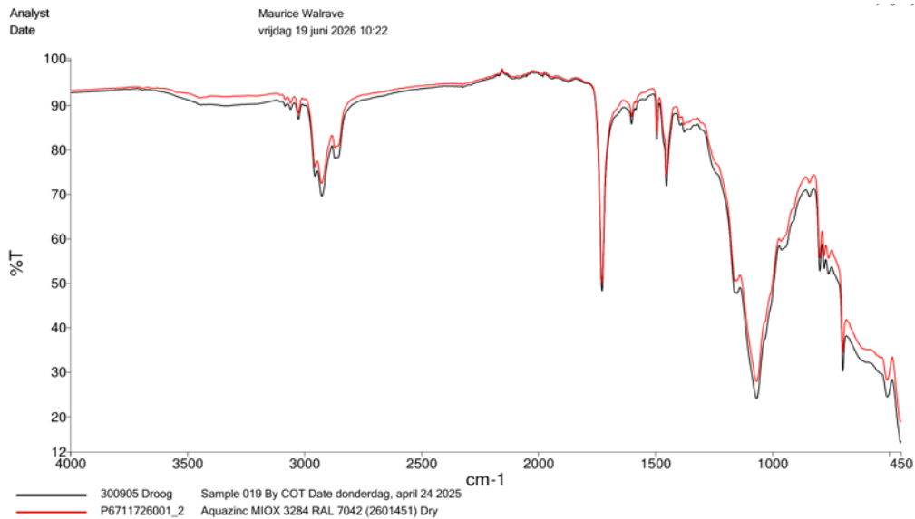
Spectra 1: Vergelijking droog C227307 F2601451
