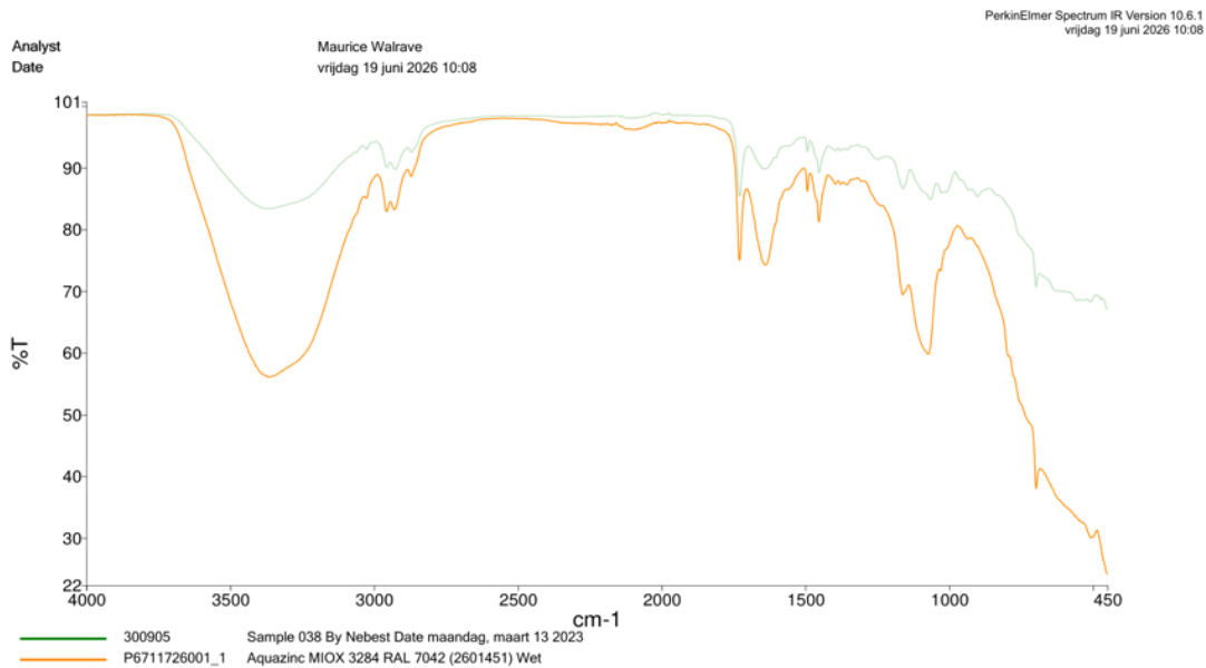
Spectra 2: Vergelijking nat C227307 F2601451
