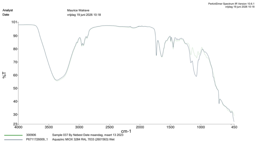
Spectra 2: Vergelijking nat C227304 F2601563
