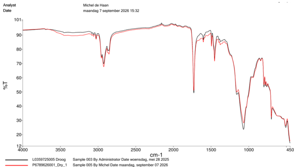
Spectra 1: Vergelijking droog C227307 F2601553
