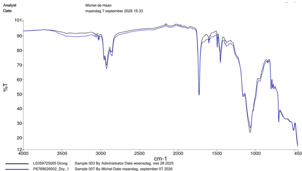
Spectra 1: Vergelijking droog C227307 F2601554
