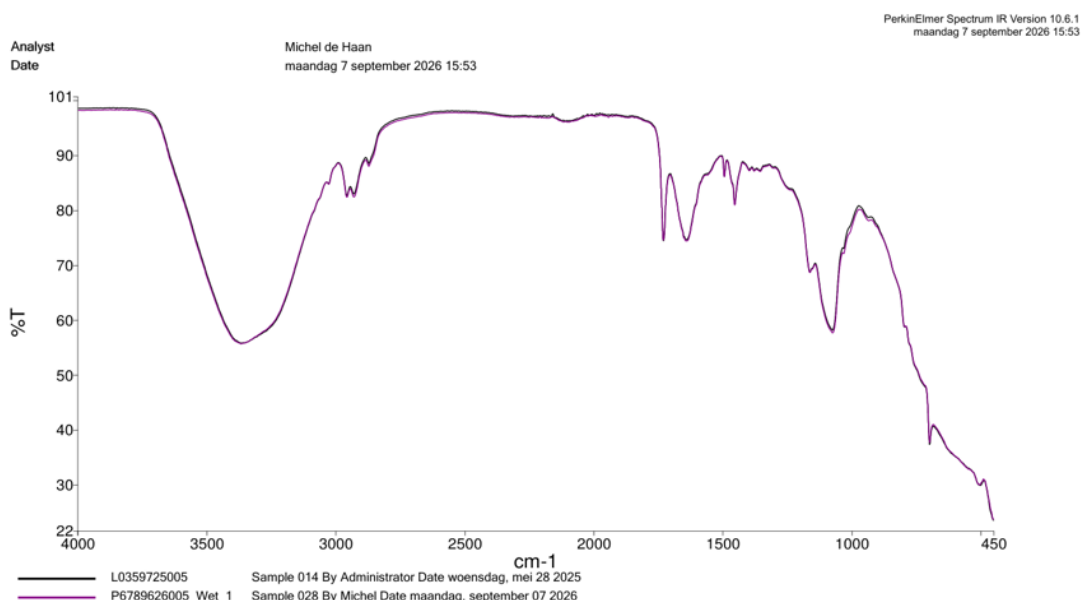
Spectra 2: Vergelijking nat C227307 F2601557
