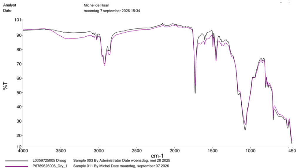
Spectra 1: Vergelijking droog C227307 F2602010
