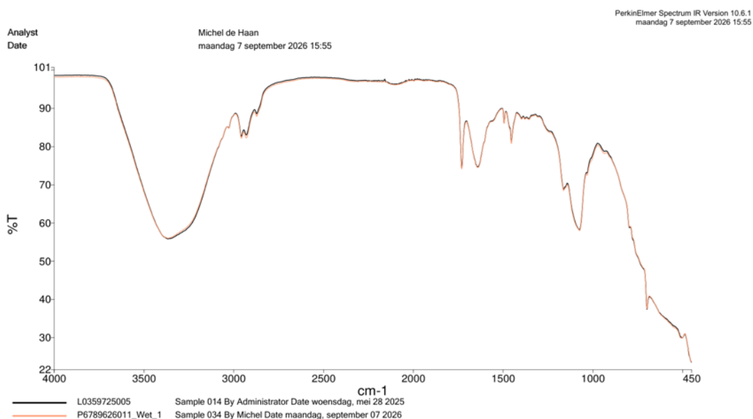
Spectra 2: Vergelijking nat C227307 F2602263
