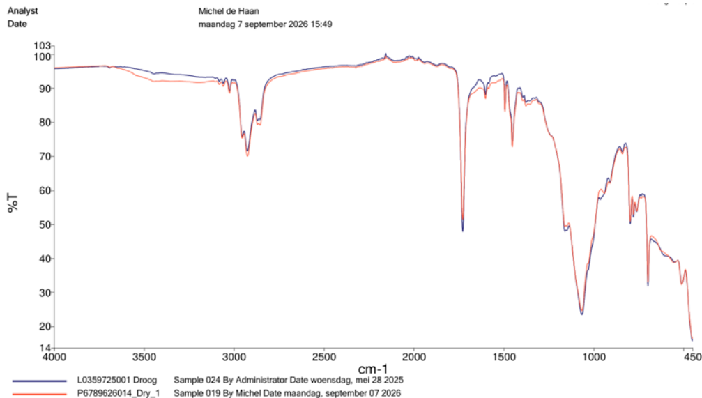
Spectra 1: Vergelijking droog C227303 F2602237
