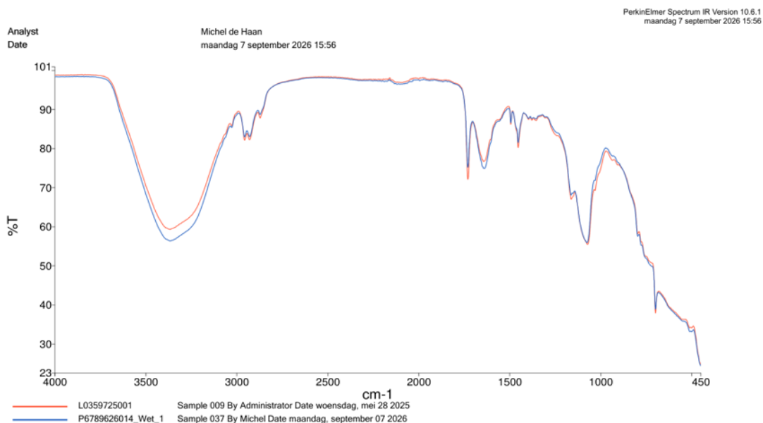
Spectra 2: Vergelijking nat C227303 F2602237
